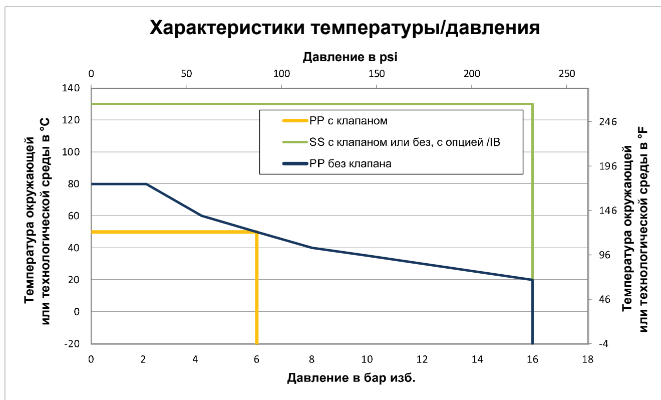
Рис. 3. Характеристики температуры/давления
