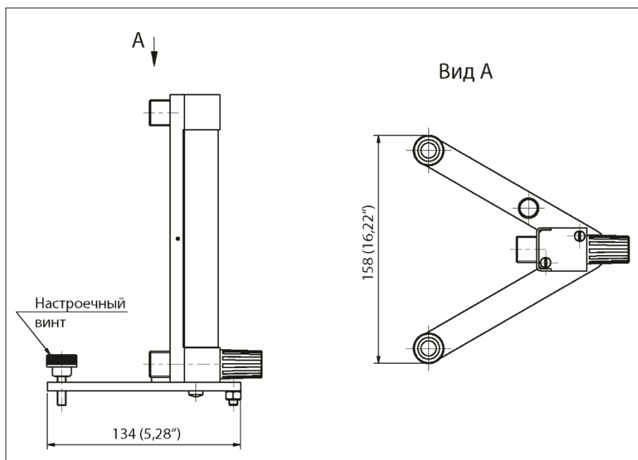
Рис. 10. Опция /QF, подставка, размеры в мм (дюймы)
