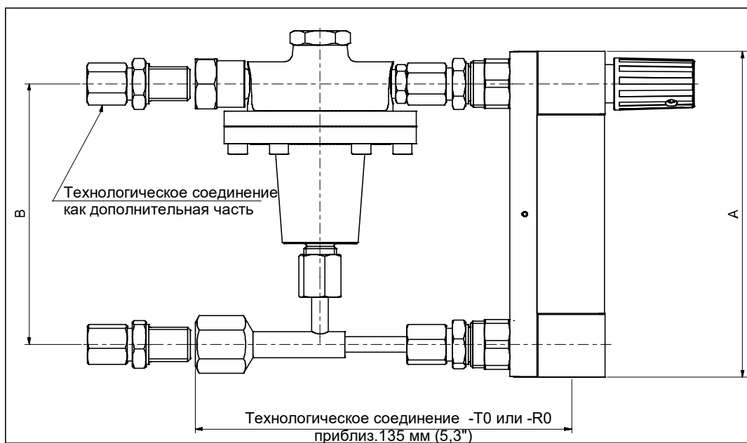
Рис. 7. Версия с выпускным клапаном и опцией контроллера выходного расхода /R3
