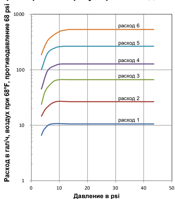
Рис. 4. Характеристики регулирования для /R1
